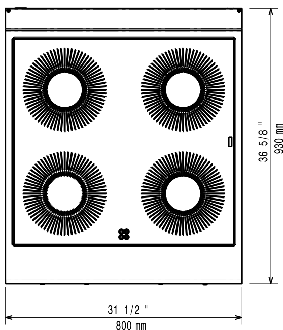
Boven aanzicht
