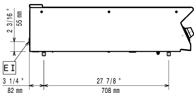
Zij aanzicht
